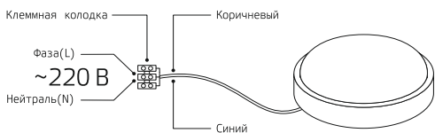
Рис. 1. Схема подключения светильника к электросети 220 В
