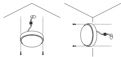
Рис. 2. Пример монтажа
